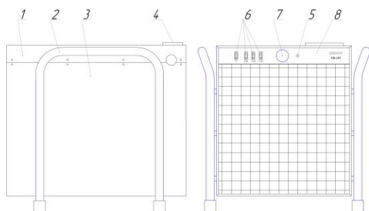
Рис.2 Общий вид электрокалорифера КЭВ-42М
