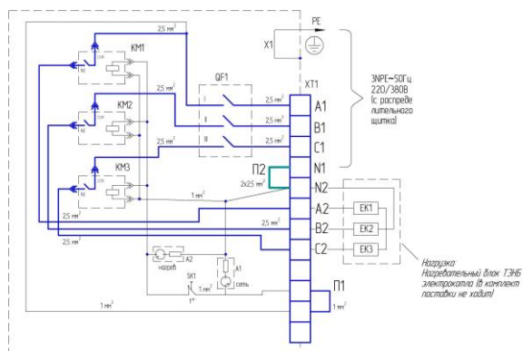
Рисунок 2 - Схема электрическая принципиальная
