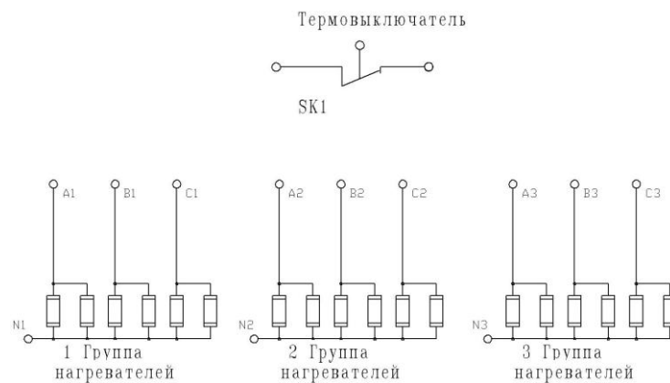
Рис.1 Схема соединений ТЭН в группы электрокалорифера СФОЦ-100
