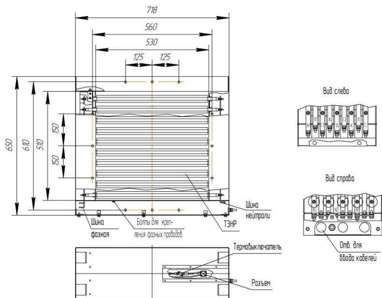
Рис.2 Общий вид электрокалорифера
