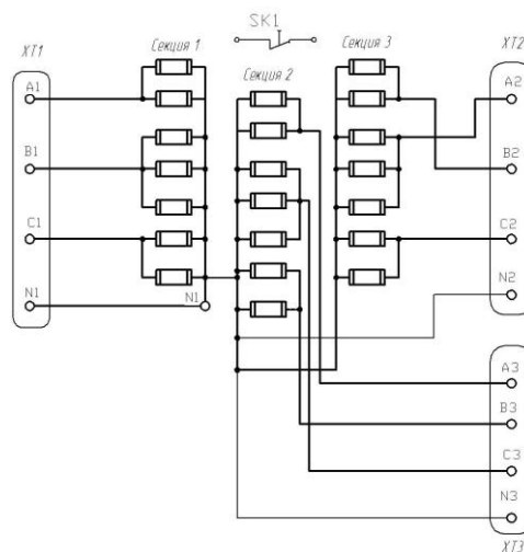
Рис.1 Схема соединений ТЭН в секции электрокалорифера
