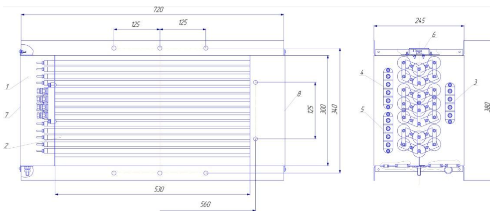
Рис.1 Схема соединений ТЭН в секции электрокалорифера
